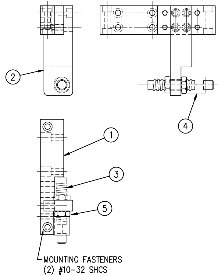
LAYOUT FOR 360 & 3600-PA PERPENDICULAR DAT
