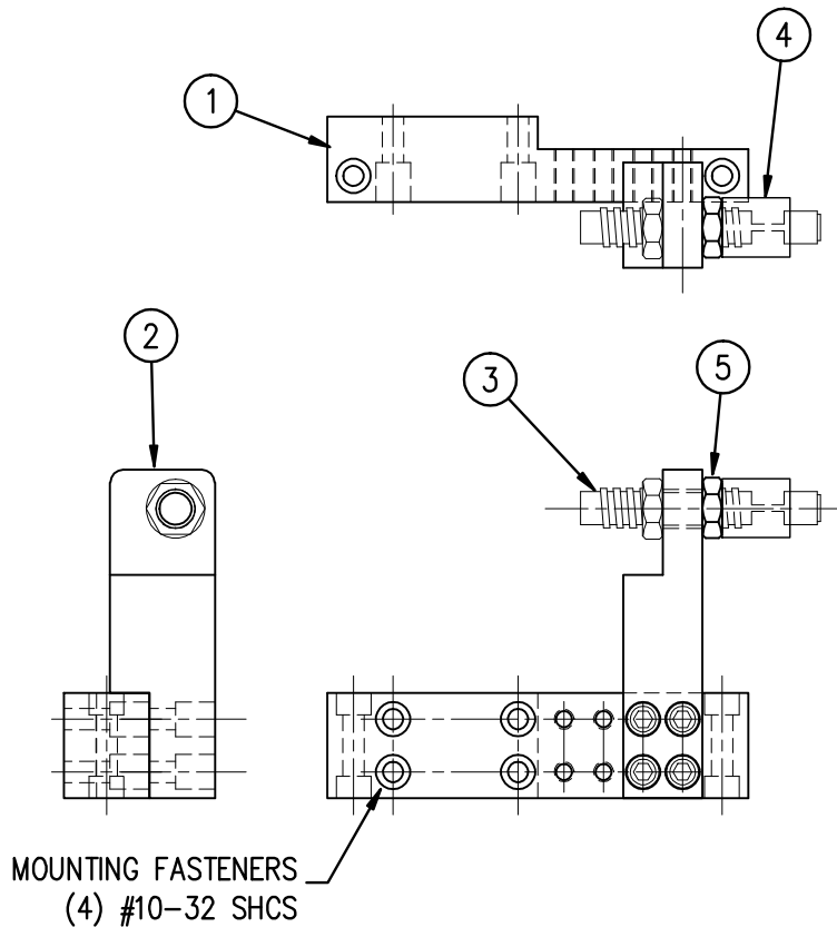
LAYOUT FOR 3600 IN-LINE DAT (REV 2)
